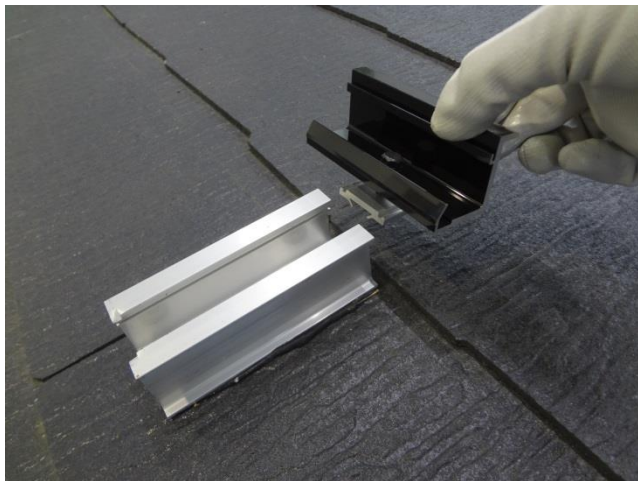
固定金具はスレート金具に差し込むだけ！
