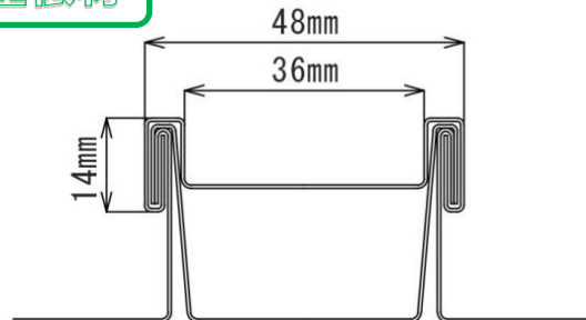
三晃金属工業株式会社製 A号瓦棒葺用金具
